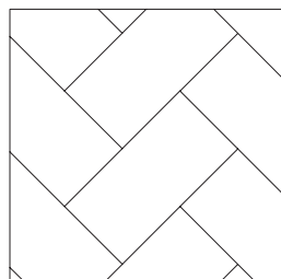
BOLDUC_AVENUE_C_30X60_2 Motif de pose chevron 45°
