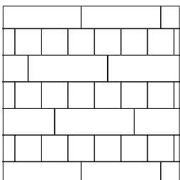
BOLDUC_AVENUE150_L_45X15_15X15_1 Motif de pose lisières alternées
