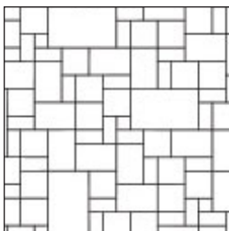
BOLDUC_RICHELIEU_M80_M2 Motif de pose modulaire 16% Richelieu M80 (80 x 163 x 325) 32% Richelieu M80 (80 x 325 x 325) 36% Richelieu M80 (80 x 325 x 488) 15% Supra Richelieu M80 (80 x 488 x 813)
