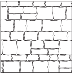
BOLDUC_VIA-APPIA80_LM_R Motif de pose lisière modulaire
