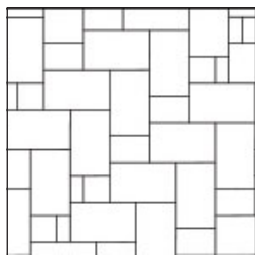
BOLDUC_RICHELIEU_M80_M1 Motif de pose modulaire 3% Richelieu M80 (80 x 163 x 325) 6% Richelieu M80 (80 x 325 x 325) 7% Richelieu M80 (80 x 325 x 488) 83% Supra Richelieu M80 (80 x 488 x 813)
