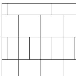
BOLDUC_AVENUE_M_ 15X30_30X30_30X60_2 Motif de pose modulaire*
