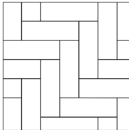
BOLDUC_AVENUE_C_15X45 Motif de pose chevron 45°
