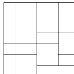
BOLDUC_AVENUE_M_ 15X30_30X30_30X60_9 Motif de pose modulaire*
