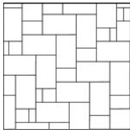
BOLDUC_CITADIN_M80_M1 Motif de pose modulaire 3% Citadin M80 (80x163x325) 6% Citadin M80 (80x325x325) 7% Citadin M80 (80x325x488) 83% Supra Citadin M80 (80x488x813)
